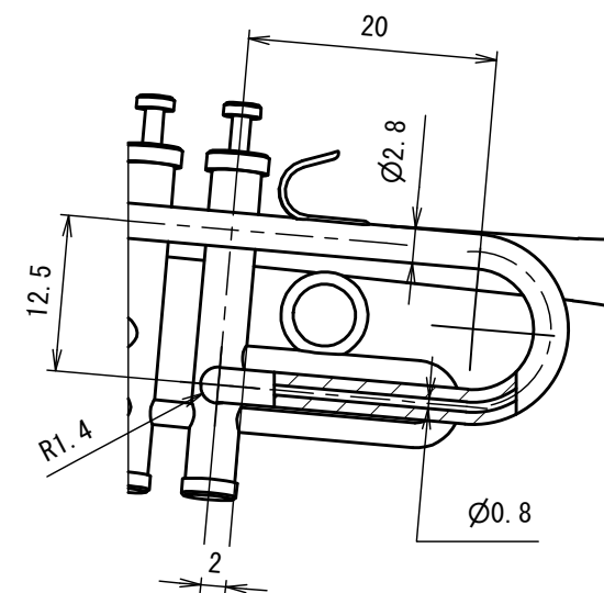
C ( 1.5 : 1 )
