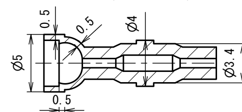
G-G ( 3 : 1 )
