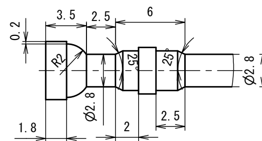
F ( 3 : 1 )
