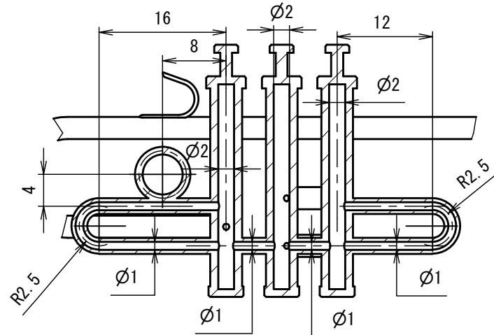
B-B ( 1.5 : 1 )
