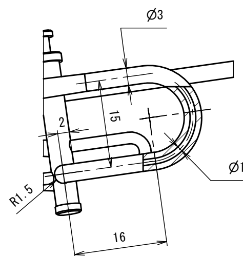
D ( 1.5 : 1 )
