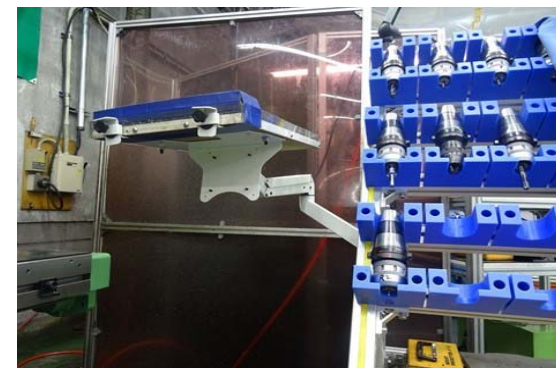
工具置きアーム(After図)
