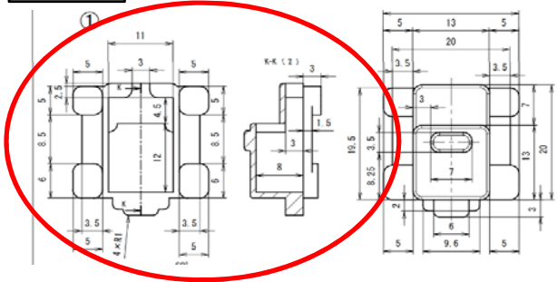
部品①
