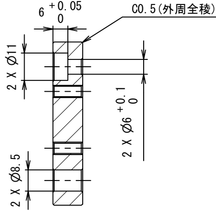
D-D ( 1 : 1.5 )
