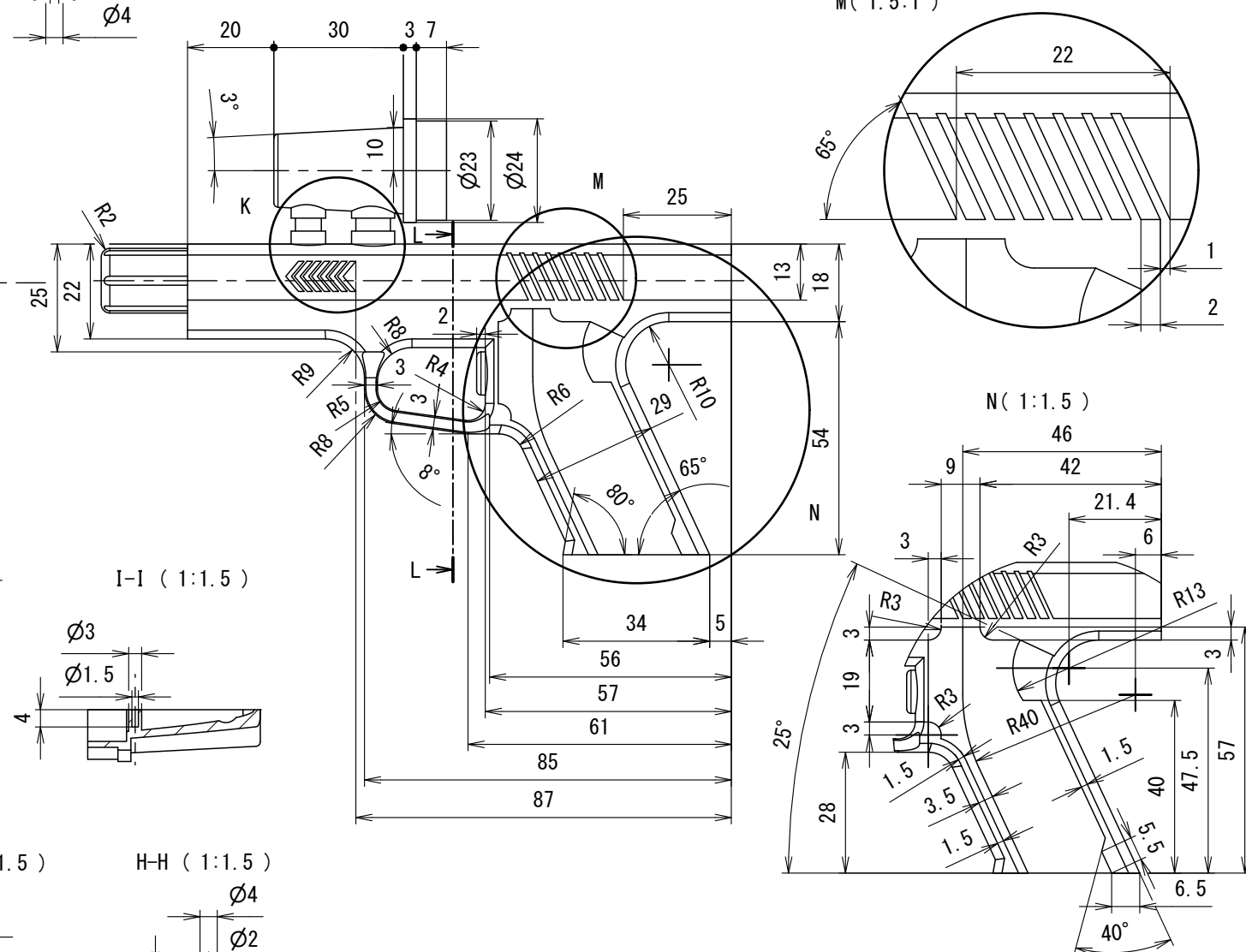
M ( 1.5:1 )
