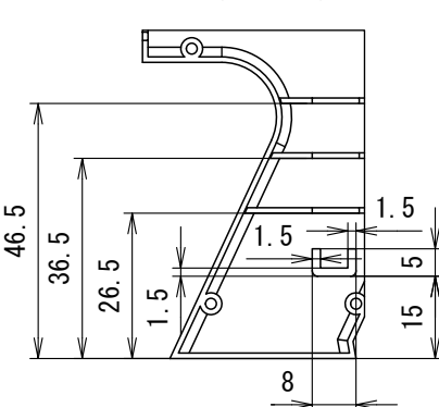
F ( 1:1.5 )
