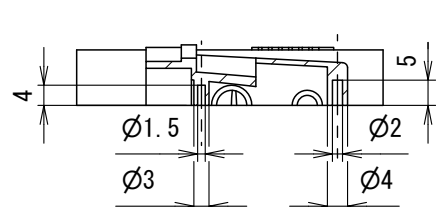
C-C ( 1:1.5 )
