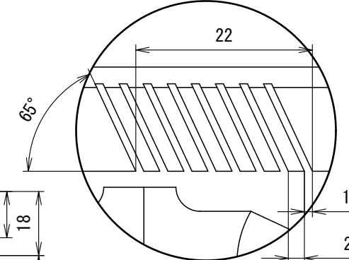
M ( 1.5:1 )
