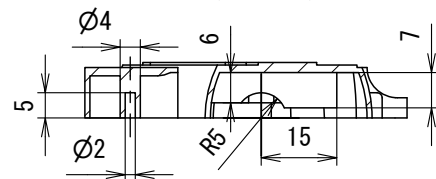
B-B ( 1:1.5 )
