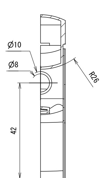
L-L ( 1 : 1 )
