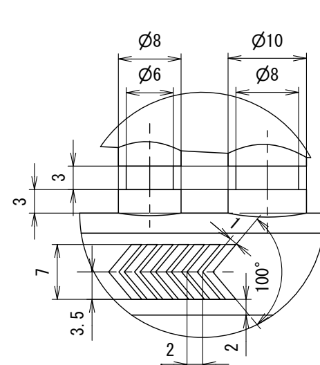
K ( 1.5:1 )
