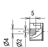
G-G ( 1:1.5 )
