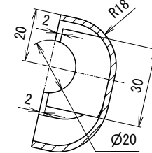
D-D (1:2)
